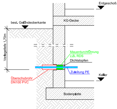
Gebäude ohne Keller Systemschnitt
