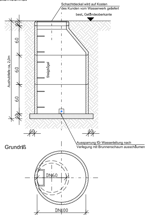
Wasserzählerschacht Systemschnitt
