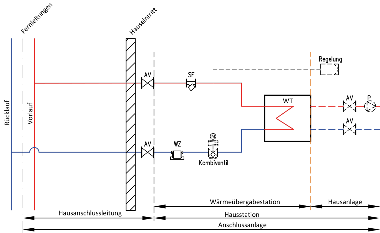
Abbildung 1: Wärmeübertragung indirekt
