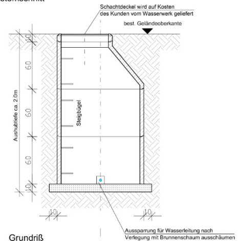
Wasserzählerschacht Systemschnitt
