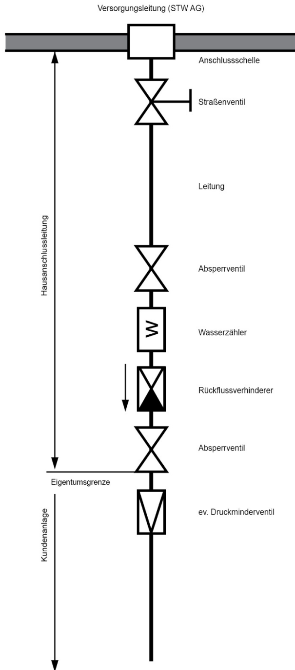
Schematische Darstellung der Anschlussleitung
